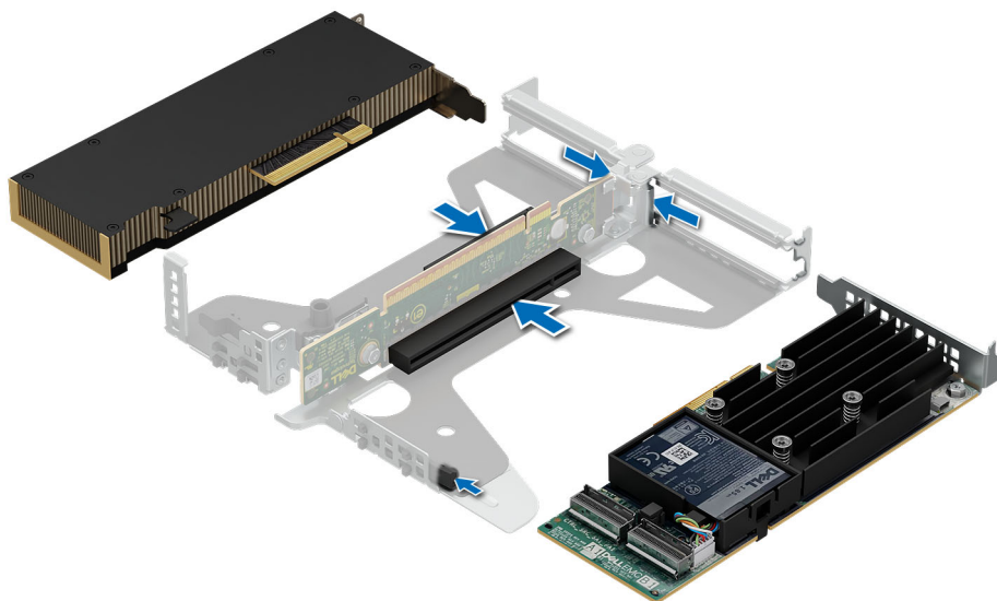
Ilustración 53. Instalación de una tarjeta de expansión en la tarjeta elevadora
