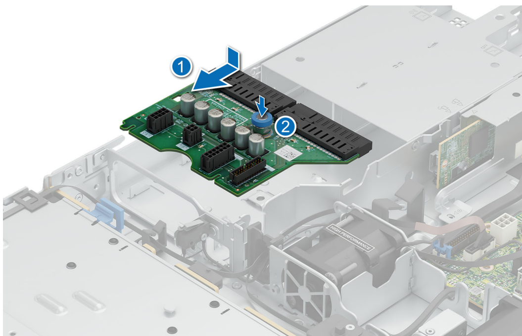
Ilustración 77. Instalación de la PIB
