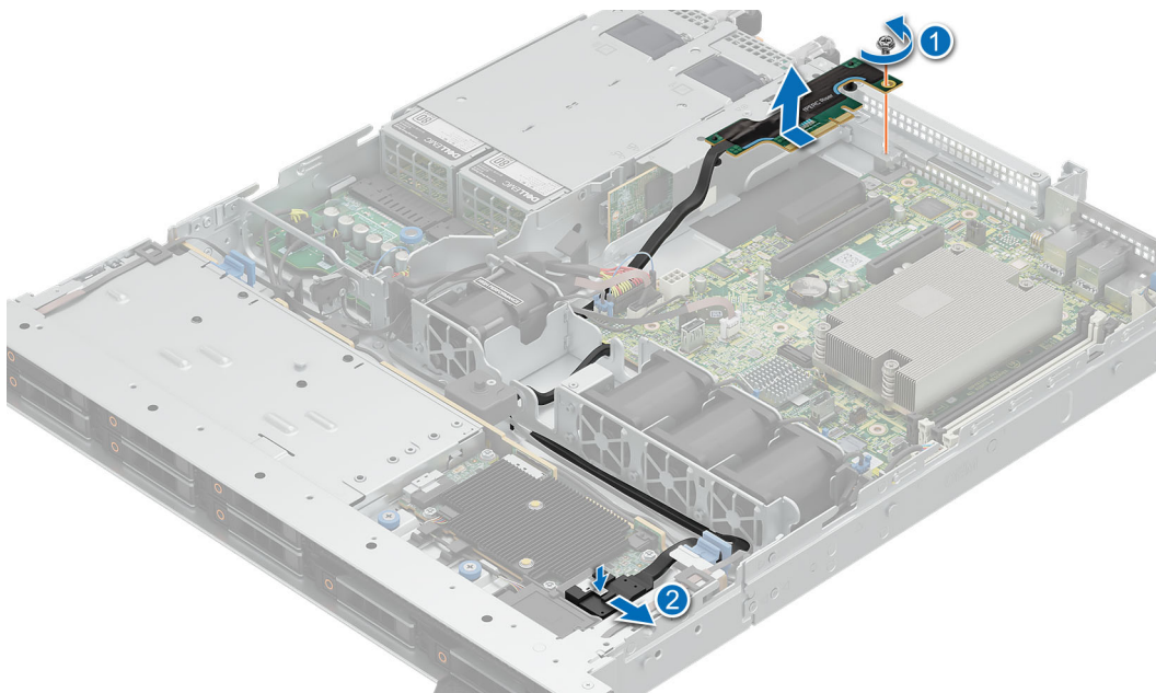
Ilustración 69. Extracción de la tarjeta elevadora de la tarjeta de PERC frontal
