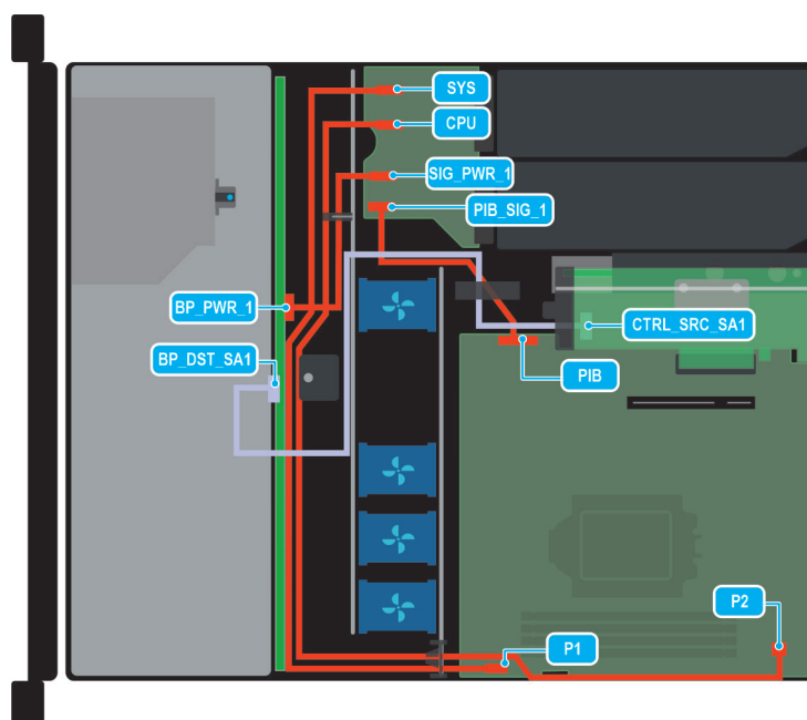
Ilustración 31. Configuración 2: 4 de SAS/SATA de 3,5 pulgadas y tarjeta PERC interna
