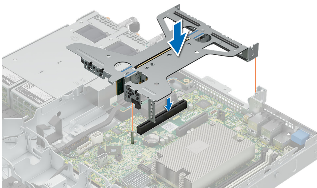
Ilustración 55. Instalación del soporte vertical
