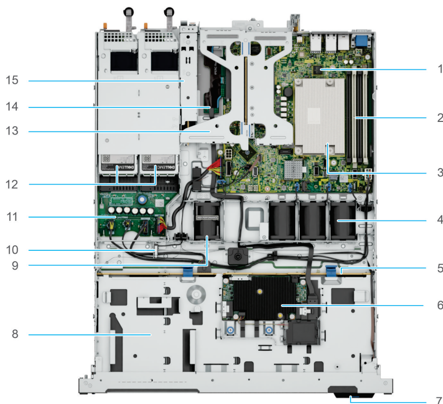
Ilustración 5. Interior del sistema
