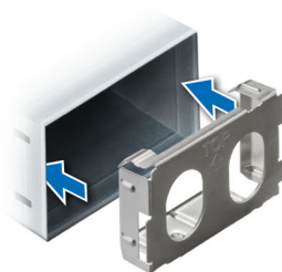
Ilustración 73. Instalación de una fuente de alimentación de relleno
