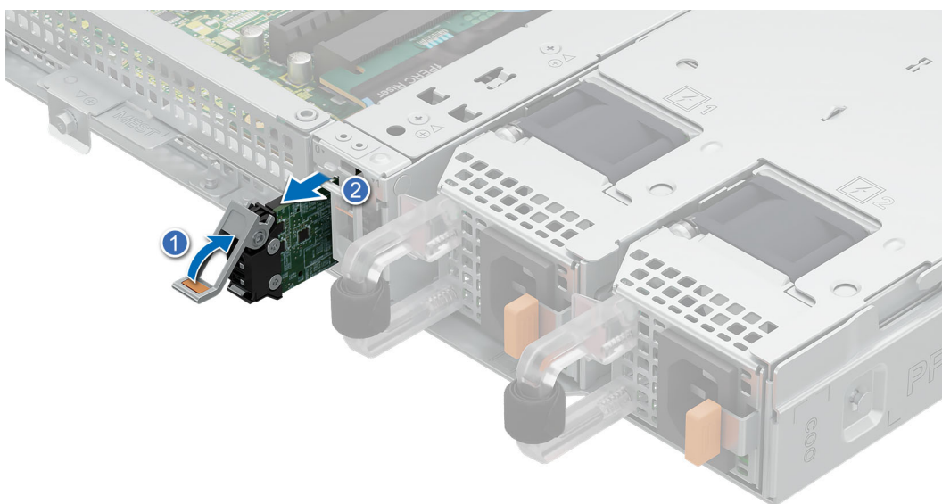
Ilustración 56. Extracción del módulo de BOSS N1 M.2
