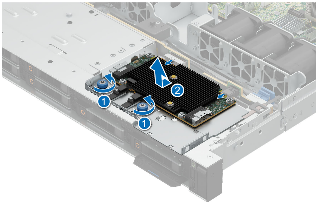
Ilustración 68. Extracción de la tarjeta de PERC frontal
