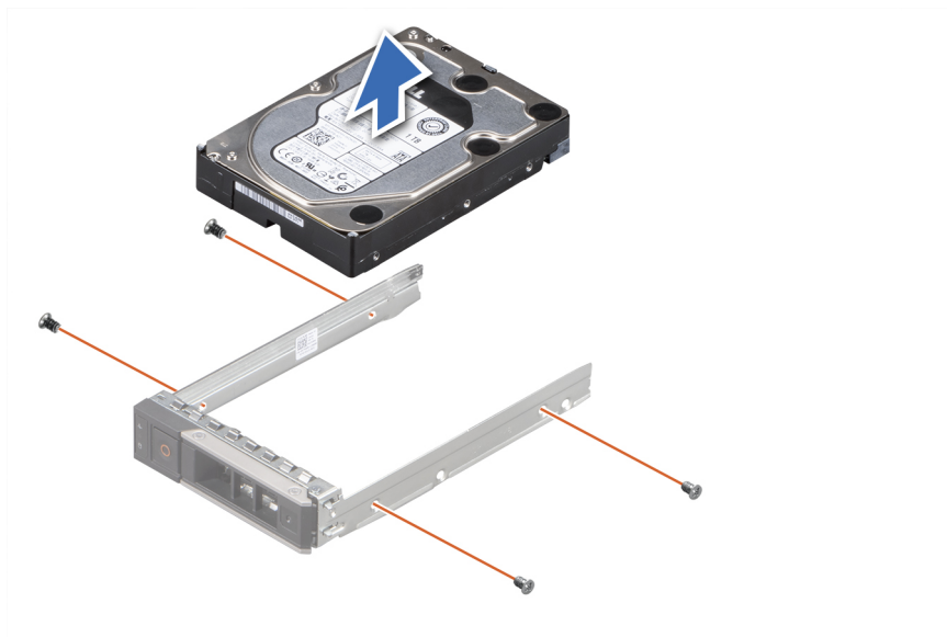
Ilustración 37. Extracción de una unidad del portaunidades
