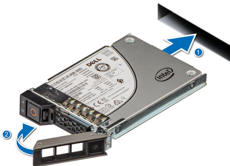
Ilustración 39. Instalación de un portaunidades
