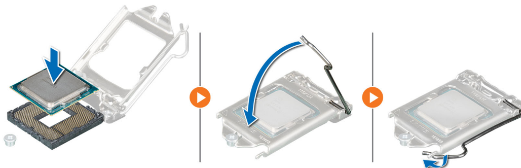
Ilustración 47. Instalación del gancho de retención
