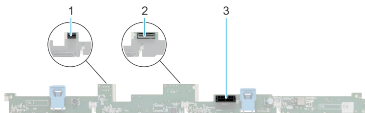
Ilustración 26. Backplane de 4 unidades SAS/SATA/SSD de 3,5 pulgadas
