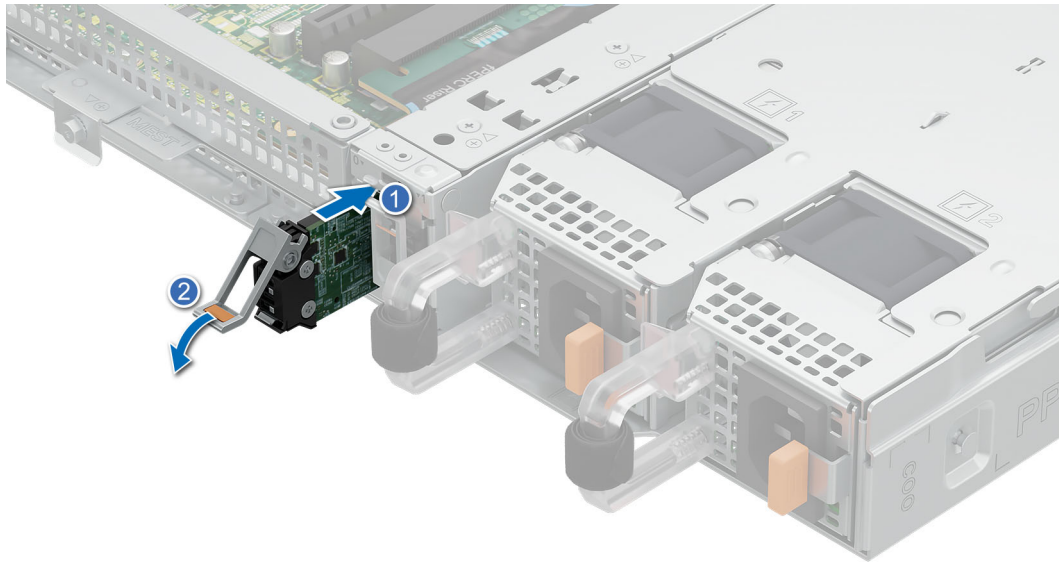
Ilustración 61. Instalación del módulo de BOSS N1 M.2
