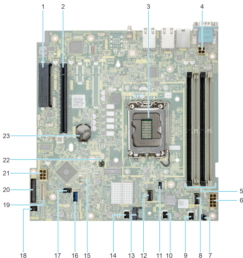
Ilustración 89. Puentes y conectores de la tarjeta madre del sistema
