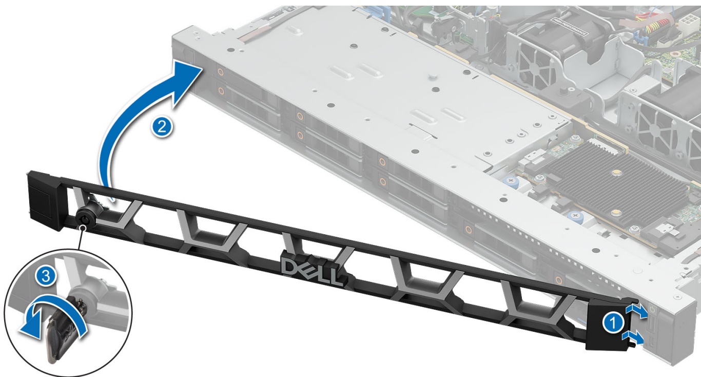
Ilustración 16. Instalación del bisel frontal
