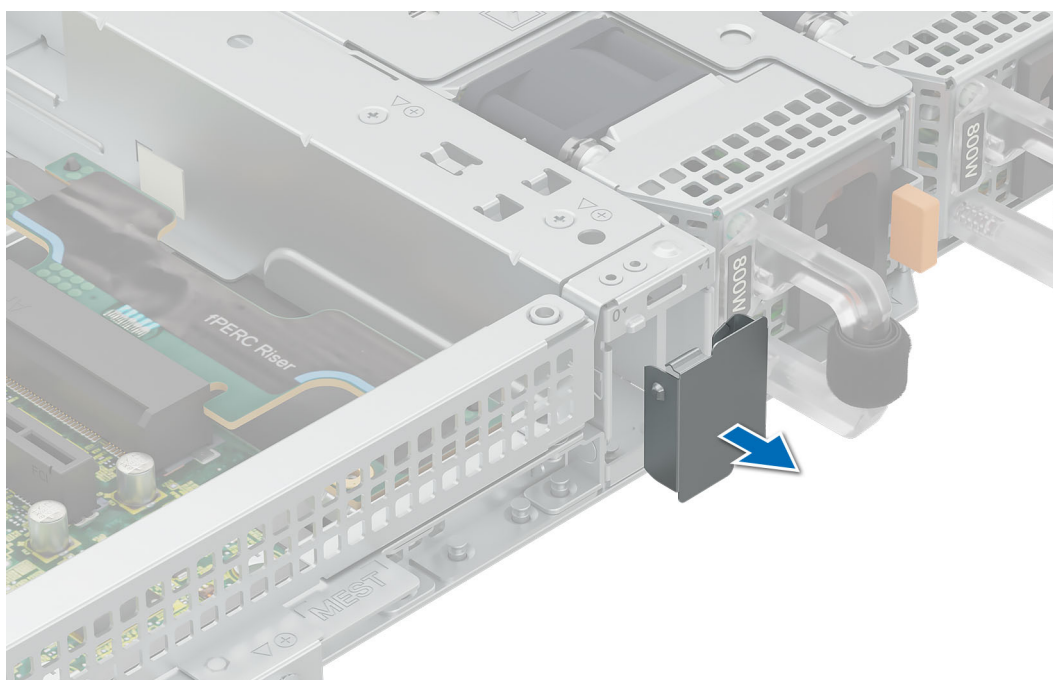
Ilustración 85. Extracción del módulo de BOSS-N1 de relleno
