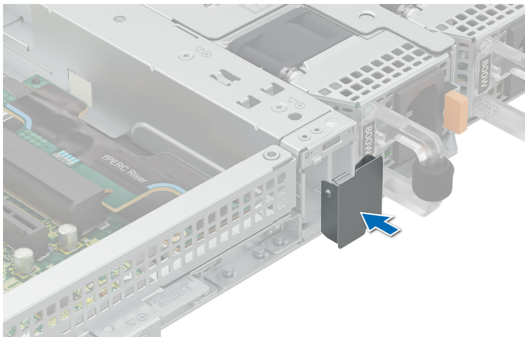
Ilustración 63. Instalación del panel de relleno de BOSS N1
