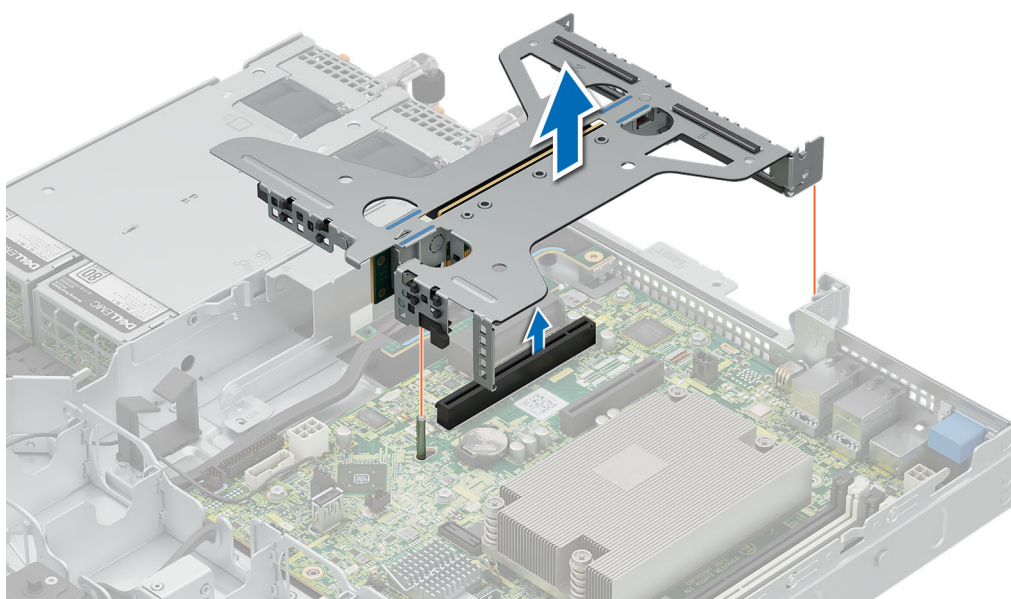
Ilustración 54. Extracción de la tarjeta elevadora
