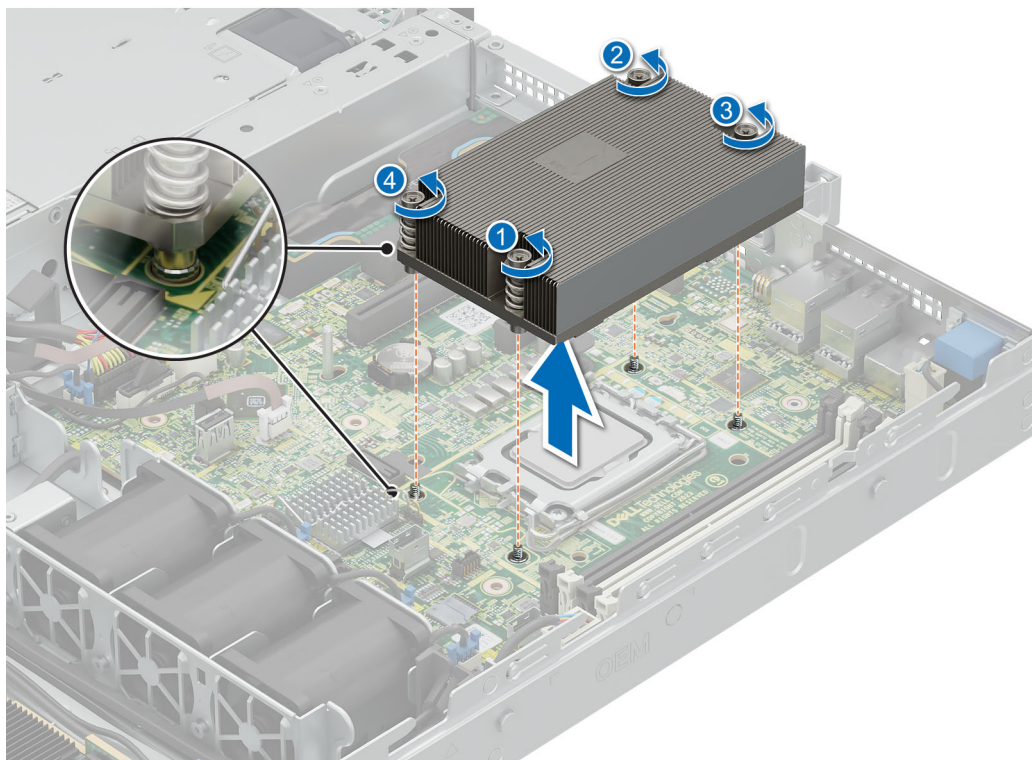
Ilustración 45. Extracción del módulo del disipador de calor
