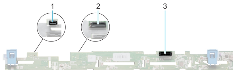
Ilustración 25. Backplane de 8 unidades SAS/SATA/SSD de 2,5 pulgadas
