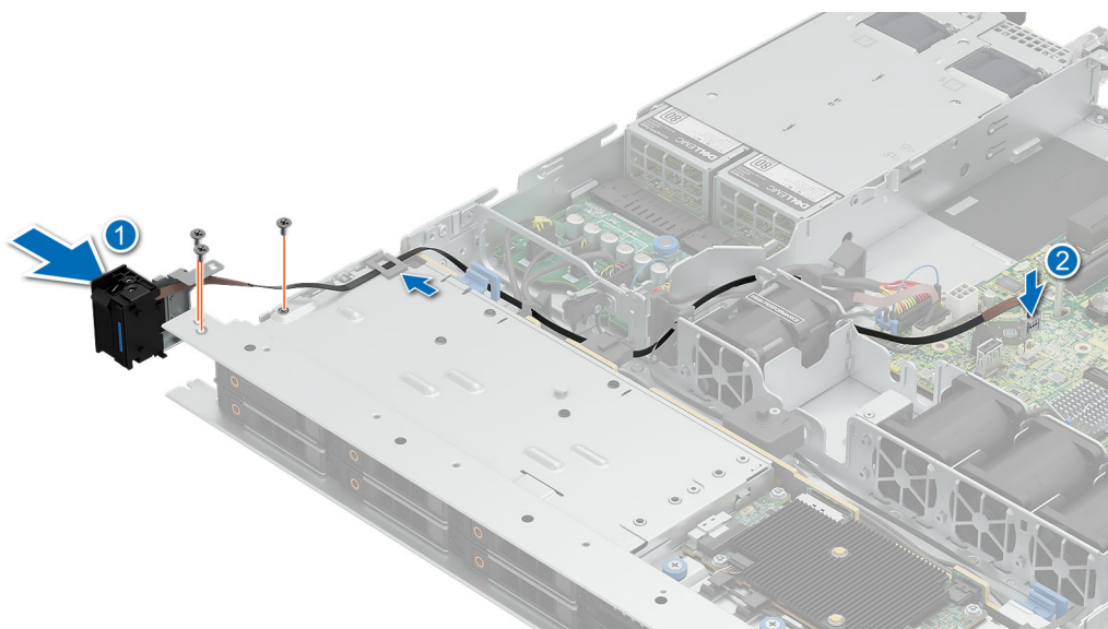
Ilustración 83. Extracción del panel de control izquierdo
