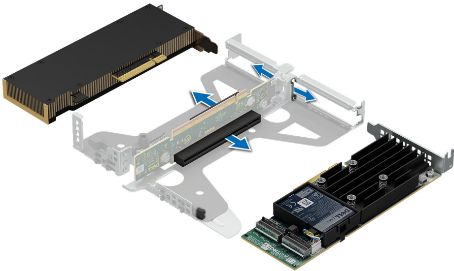
Ilustración 51. Extracción de una tarjeta de expansión de la tarjeta elevadora
