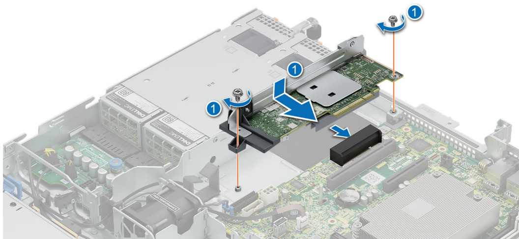
Ilustración 67. Instalación de la tarjeta PERC interna
