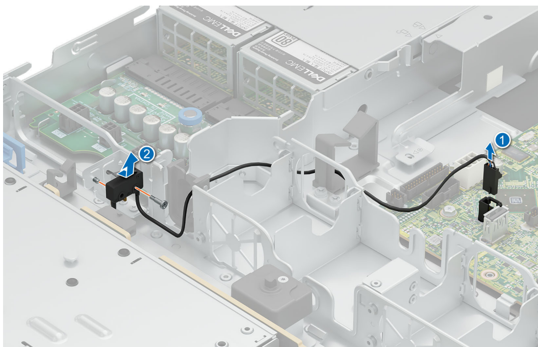
Ilustración 23. Extracción del interruptor de intrusiones
