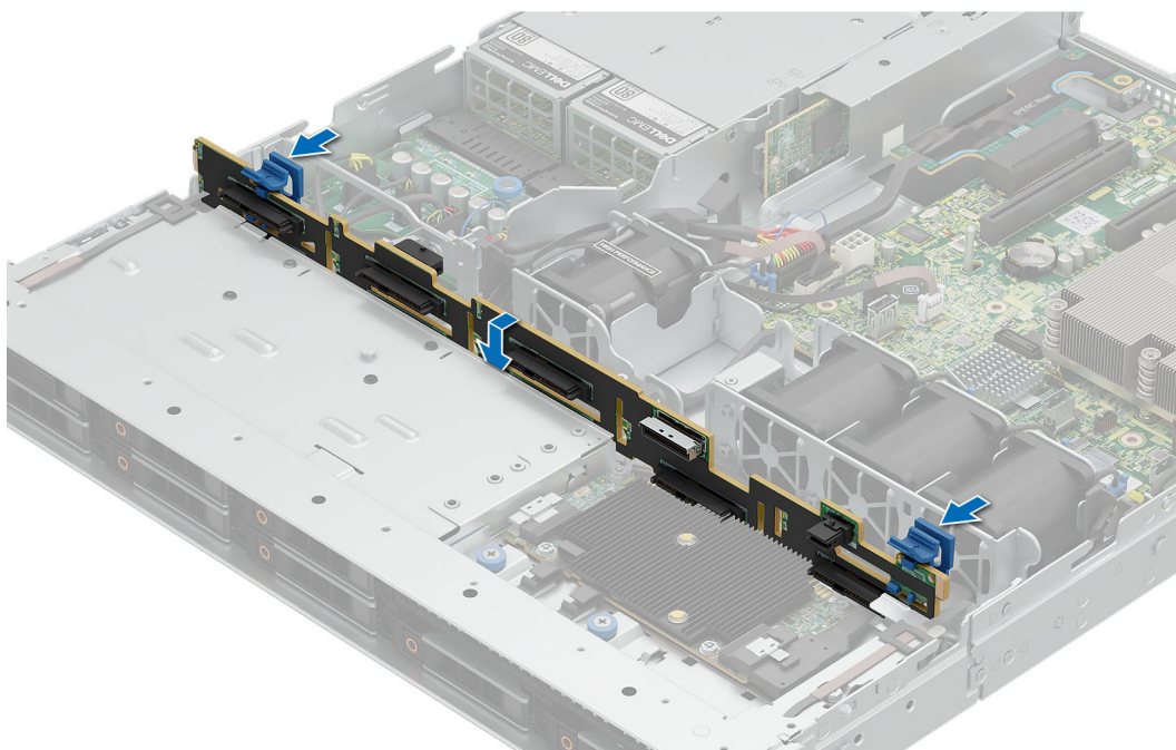
Ilustración 28. Instalación del backplane de la bahía de unidad frontal
