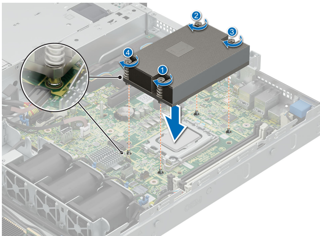
Ilustración 50. Instalación del disipador de calor
