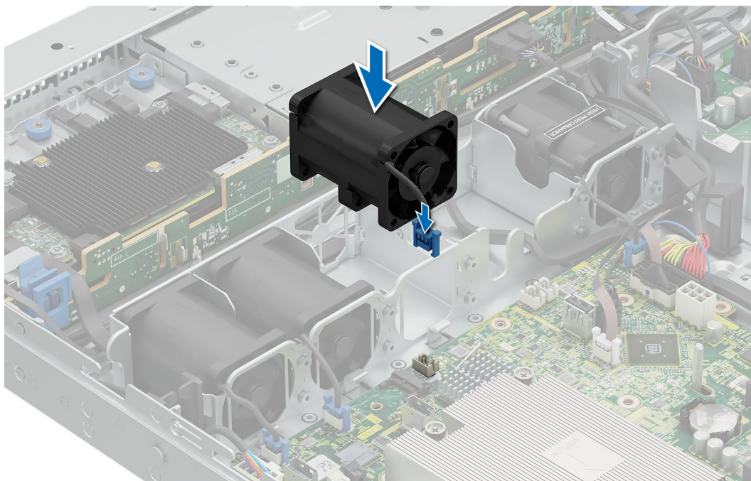
Ilustración 22. Instalación de un ventilador
