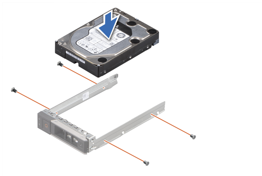
Ilustración 38. Instalación de una unidad en el portaunidades
