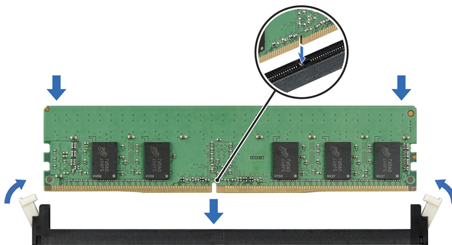
Ilustración 44. Instalación de un módulo de memoria
