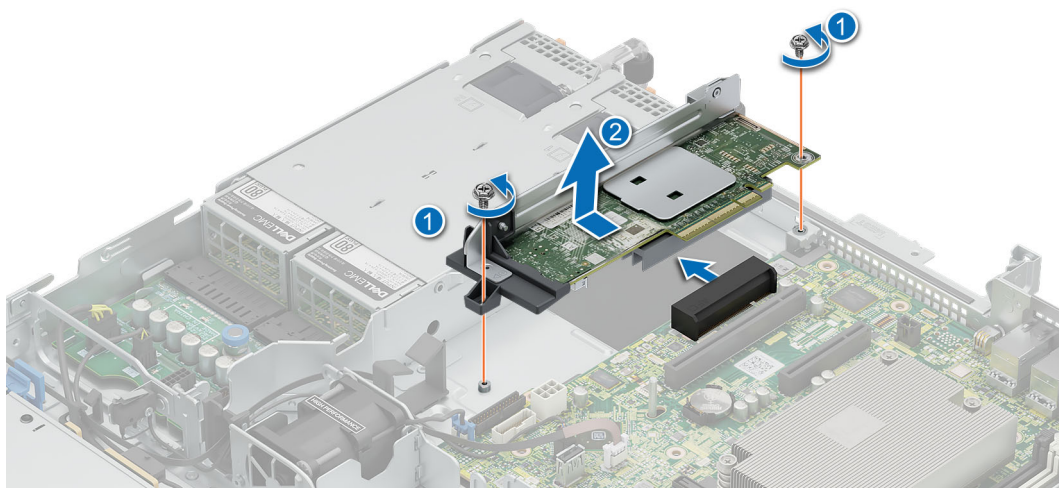
Ilustración 66. Extracción de la tarjeta PERC interna
