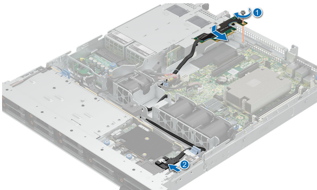
Ilustración 71. Instalación de la tarjeta elevadora de PERC frontal
