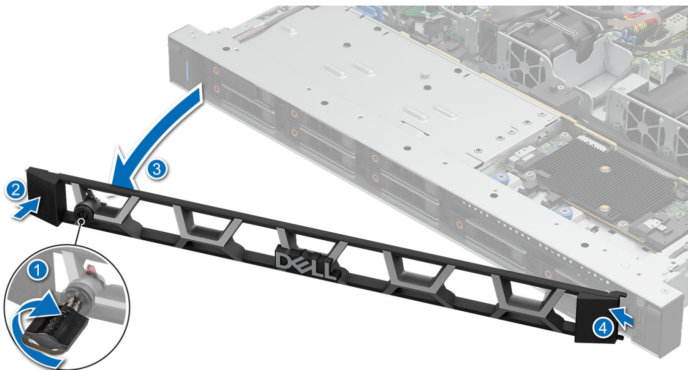
Ilustración 15. Extracción del bisel frontal
