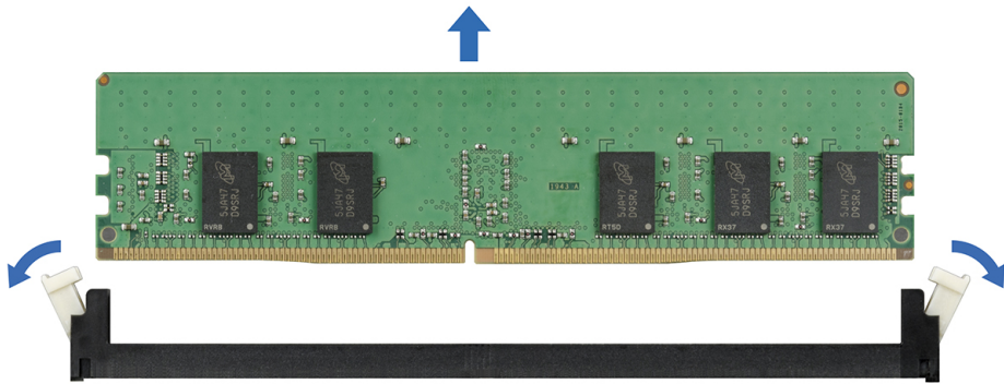
Ilustración 43. Extracción de un módulo de memoria
