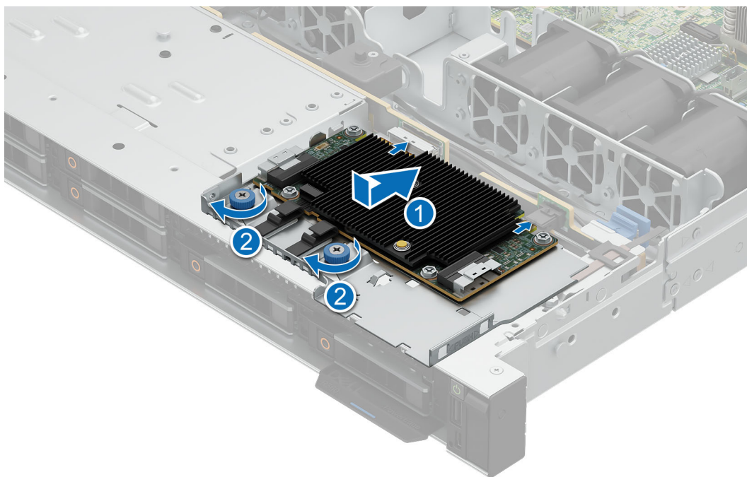
Ilustración 70. Instalación del módulo de PERC frontal
