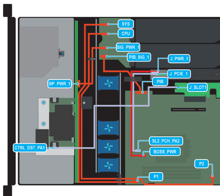
Ilustración 30. Configuración 1: SAS/SATA de 4 x 3,5 pulgadas y fPERC con BOSS N1 (opcional)
