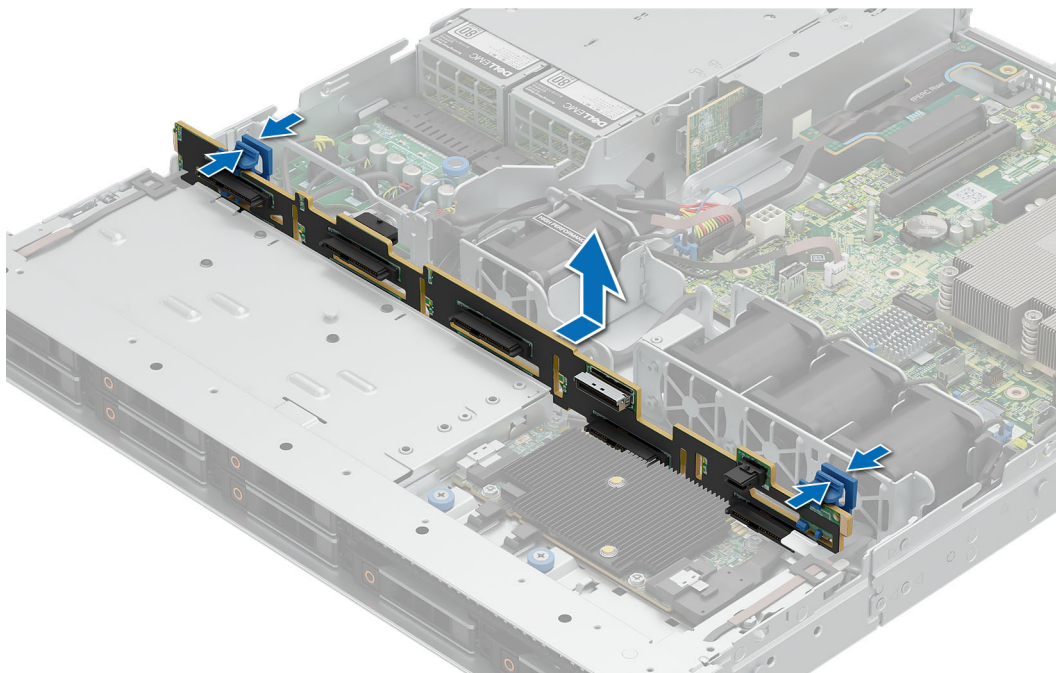
Ilustración 27. Extracción del backplane de la bahía de unidad frontal
