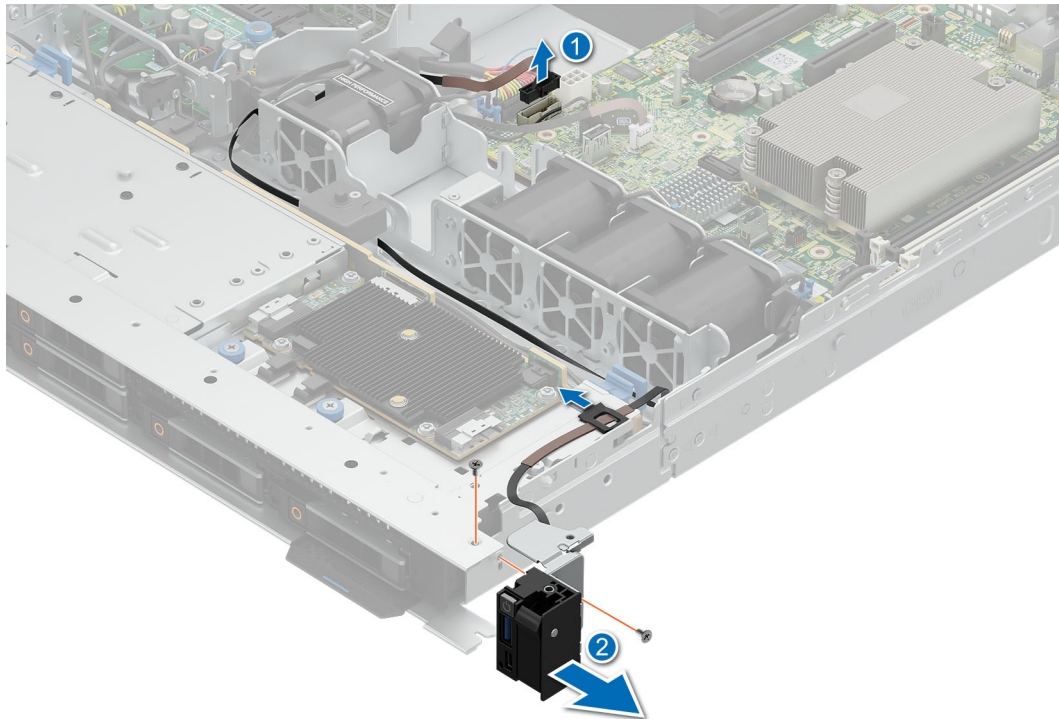
Ilustración 81. Extracción del panel de control derecho
