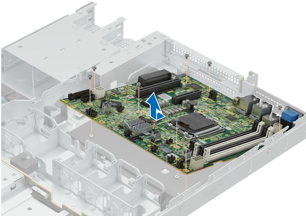
Ilustración 78. Extracción de la tarjeta madre
