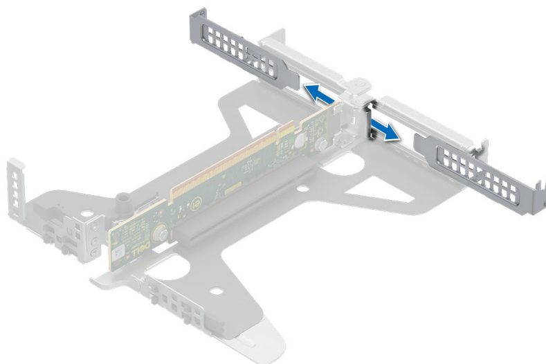
Ilustración 52. Extracción del soporte de relleno de la tarjeta elevadora
