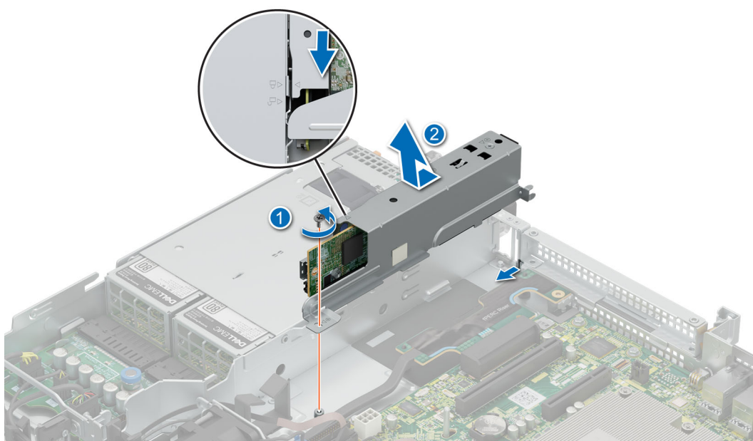
Ilustración 57. Extracción de la canastilla de BOSS N1
